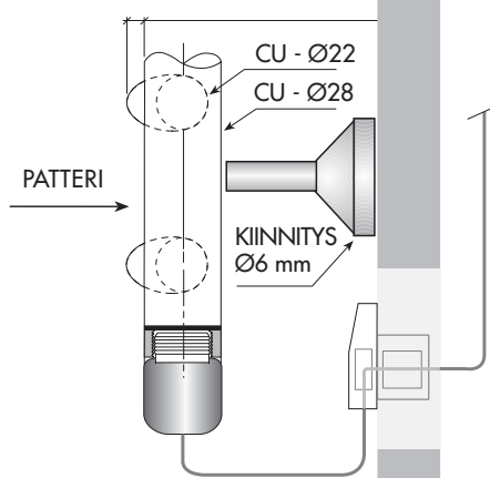
Puolikiinteä asennus
